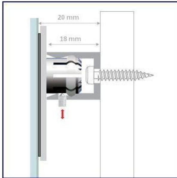
Blinde bevestiging
